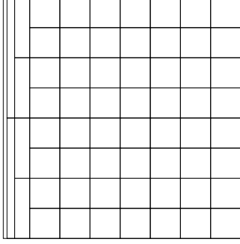
FIG. 13. The tiling s_{64} .
